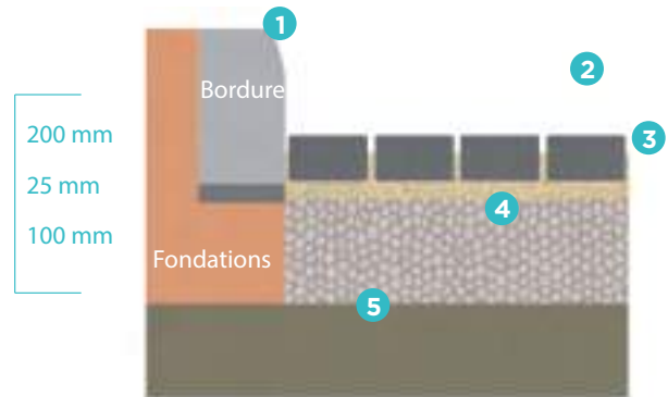
Exemple de blocage des rives à l'aide de bordures et/ou caniveaux
