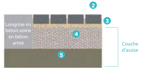
Exemple de blocage des rives au moyen d'une longrine en béton
