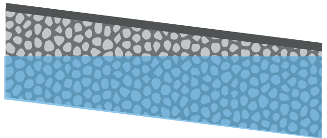
Compartment de chaussée à structure réservoir
